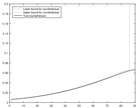
(d) \beta = .95 , using Corollaries 3 and 4.
